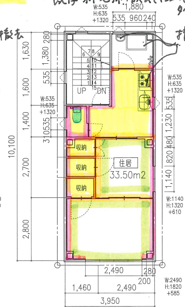
5階 〈住居〉
