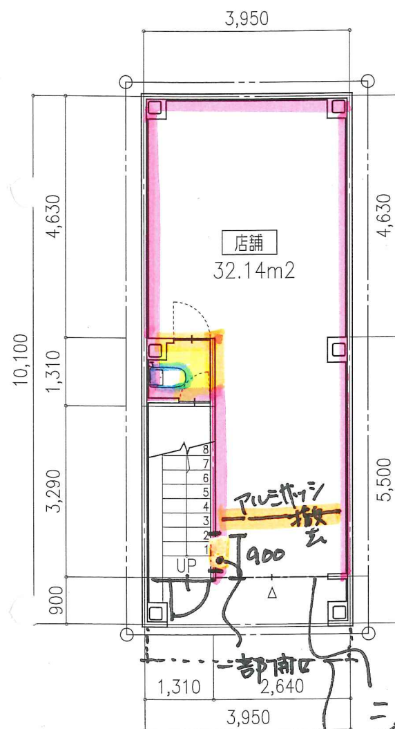
1階 〈店舗〉
