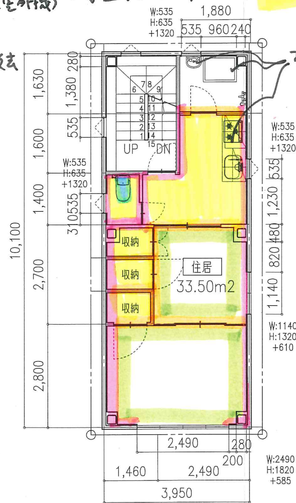
4階 〈住居〉
